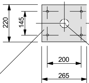
Монтажное основание
